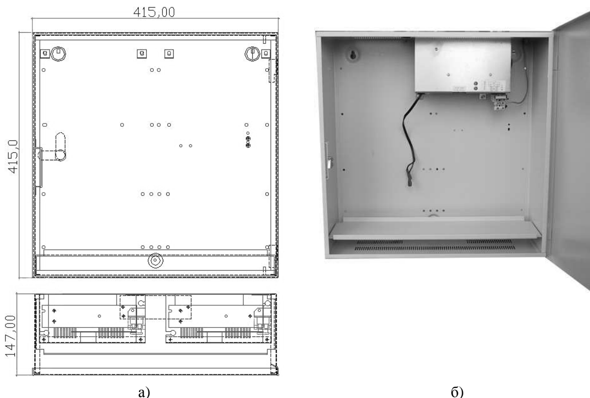
Рисунок 1.1 – Внешний вид ИБП Штиль PS4802E а) габаритные размеры; б) внешний вид
